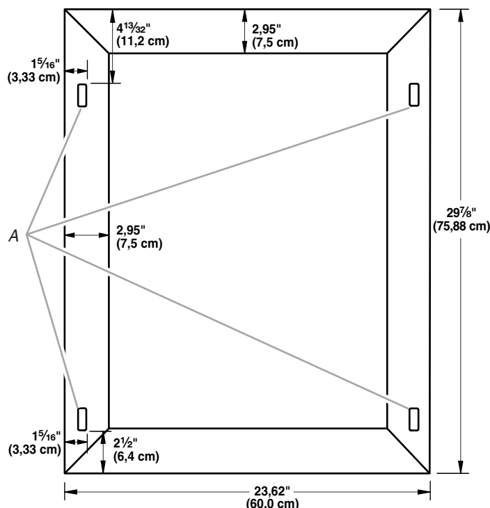
A. Ubicaciones de los ganchos del revestimiento
