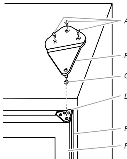
A. Vis (3) B. Charnière supérieure C. Rondelle D. Cale d'espacement supérieure E. Porte F. Cadre décoratif
